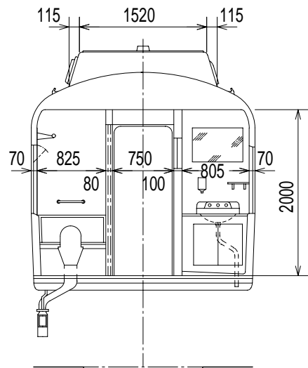
断面視 f-f
