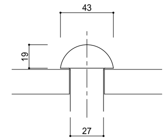
呼び径 43 (2欄) 長さ 38~140
