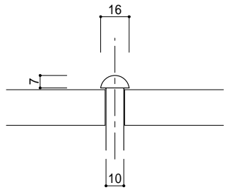
呼び径 16 (1欄) 長さ 10~50
