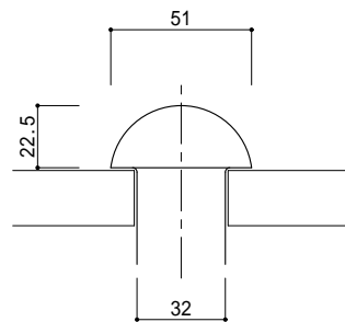
呼び径 51 (3欄) 長さ 45~160
