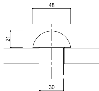
呼び径 48 (1欄) 長さ 40~150
