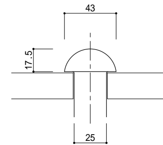
呼び径 43 (3欄) 長さ 36~130
