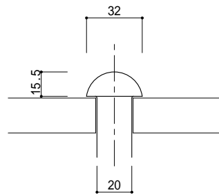
呼び径 32 (1欄) 長さ 24~110
