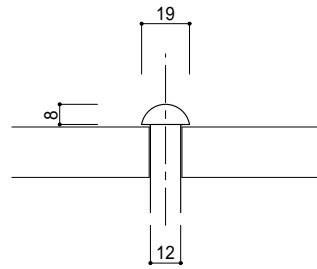
呼び径 19 (1欄) 長さ 12~60
