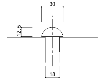
呼び径 30 (2欄) 長さ 20~90
