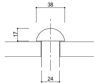
呼び径 38 (1欄) 長さ 32~130
