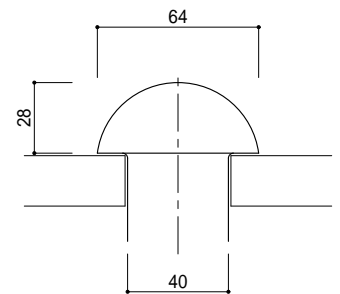
呼び径 64 (2欄) 長さ 60~190
