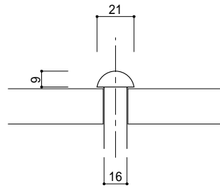
呼び径 21 (3欄) 長さ 14~65
