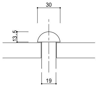
呼び径 30 (3欄) 長さ 22~100
