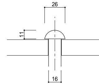
呼び径 26 (1欄) 長さ 18~80
