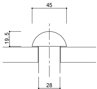
呼び径 45 (3欄) 長さ 38~140
