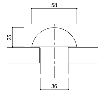
呼び径 58 (1欄) 長さ 50~180
