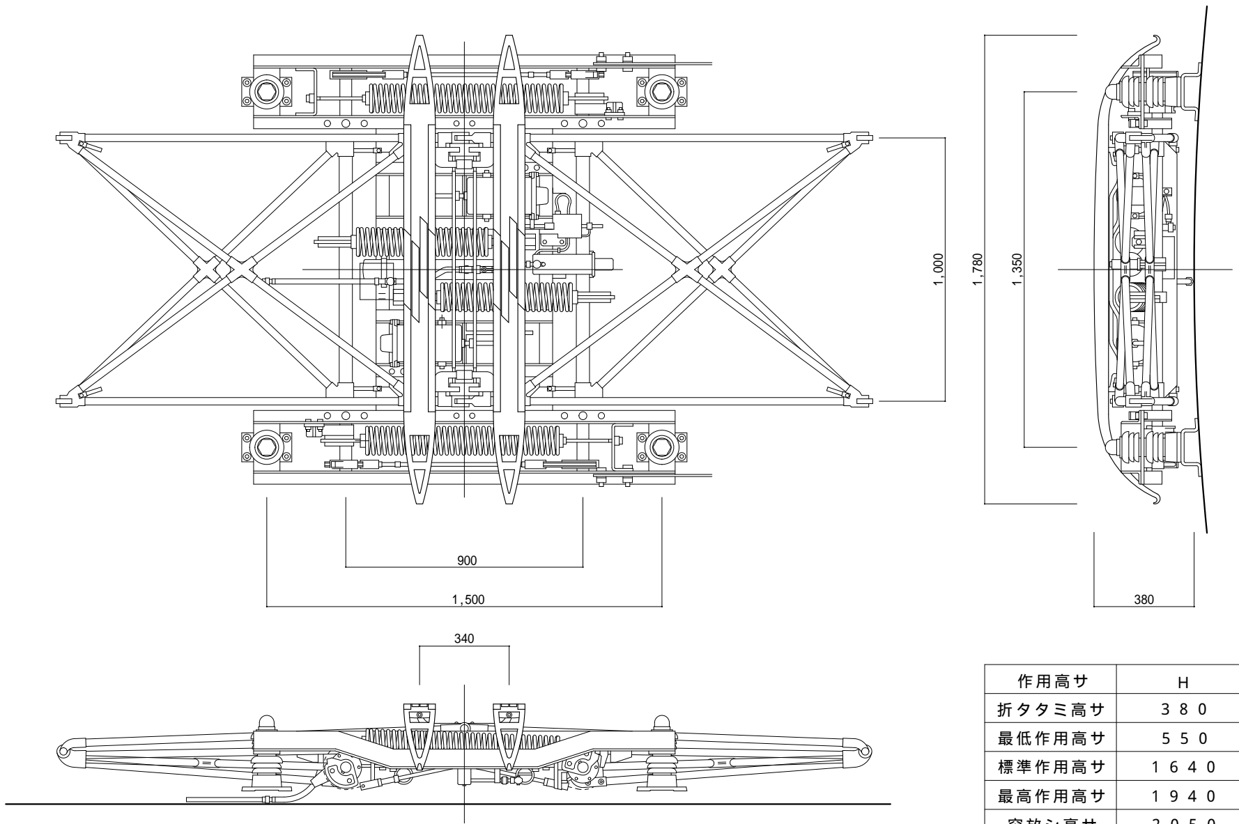
PS10A型パンタグラフ
