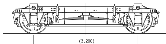
ケ'ルリツ折衷台車
