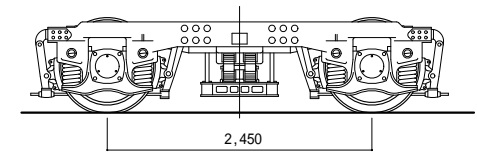
TR 4 7 (軽量軸箱)
