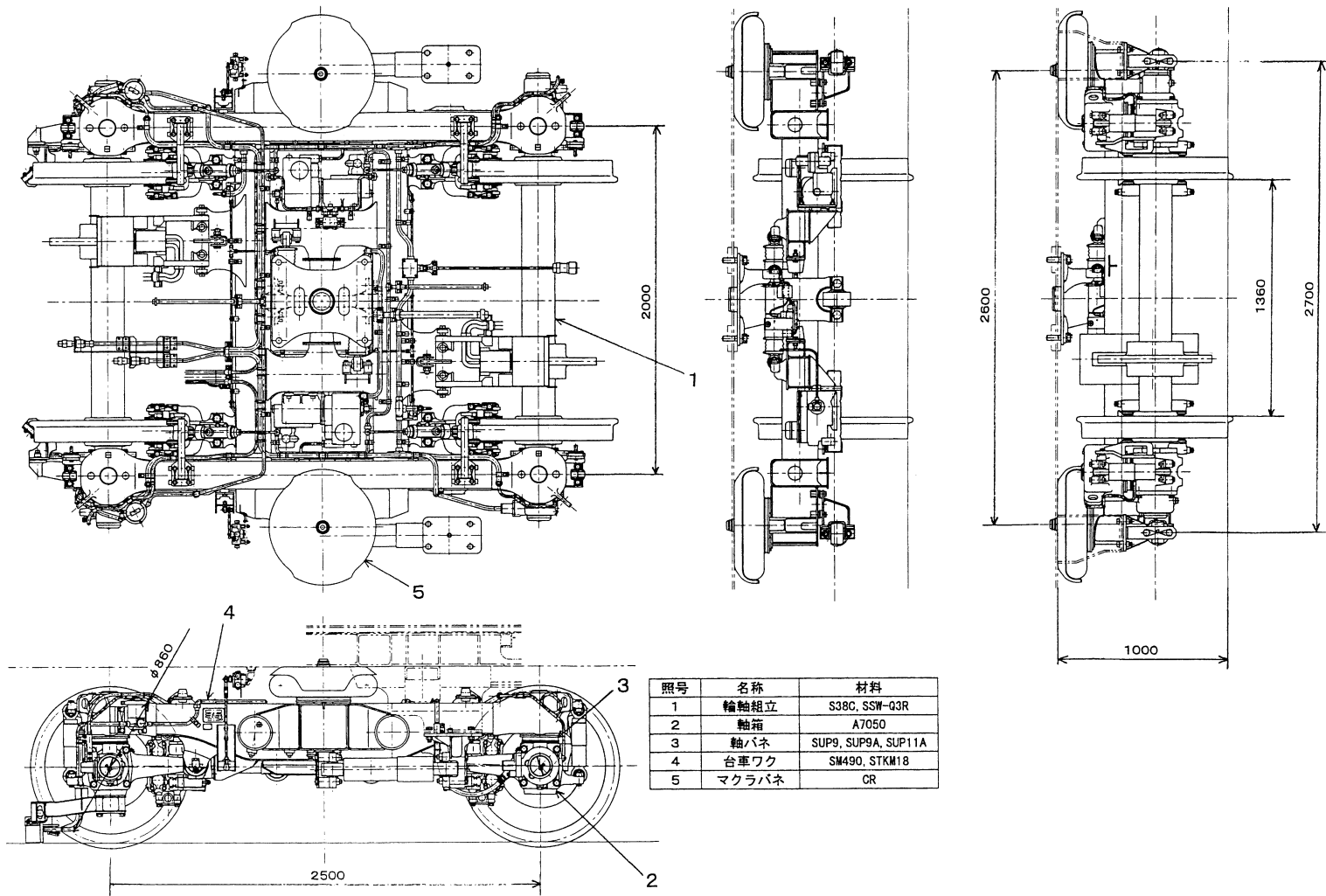
図19 付随台車 (TR7002-G1)
