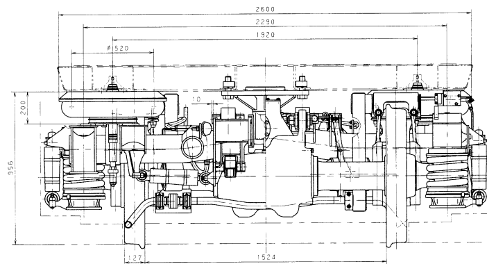
図5 駆動台車組立 (TS-1022)
