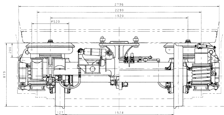
図7 付随台車組立 (TS-1025)
