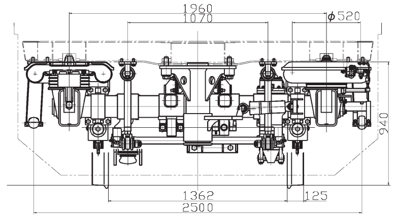
图 6 動台車 (22600 形、22800 形)
