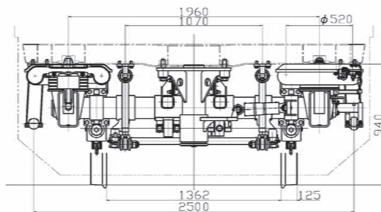
図7 付随台車 (22700形、22900形)
