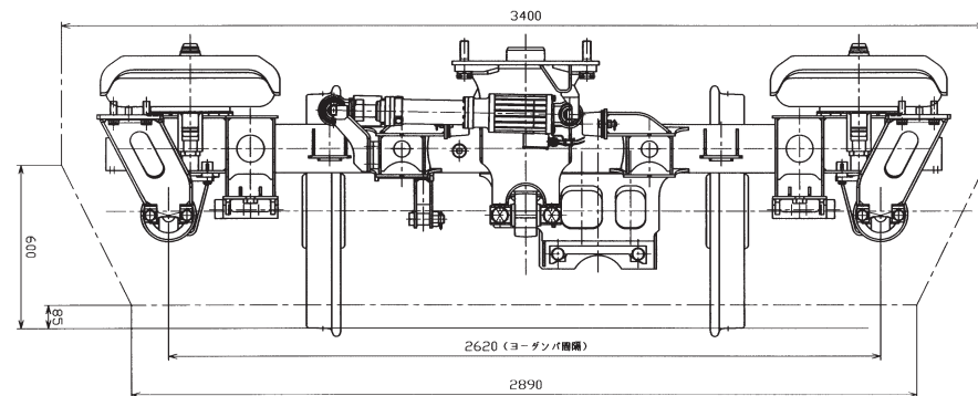
図9 動台車 (DT209)
