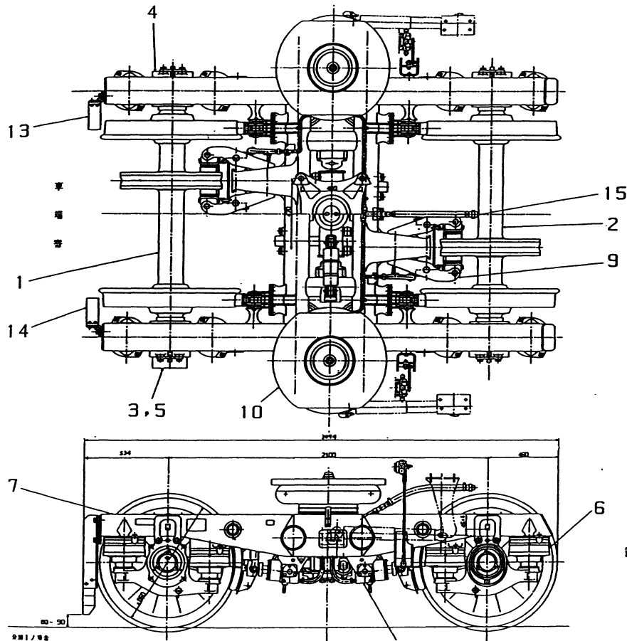
図8 付随台車(C-TR241)
