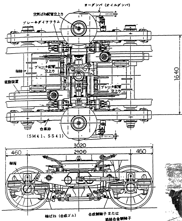
図 11 台車 (DT56)
