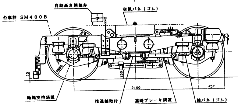
図4 台車
