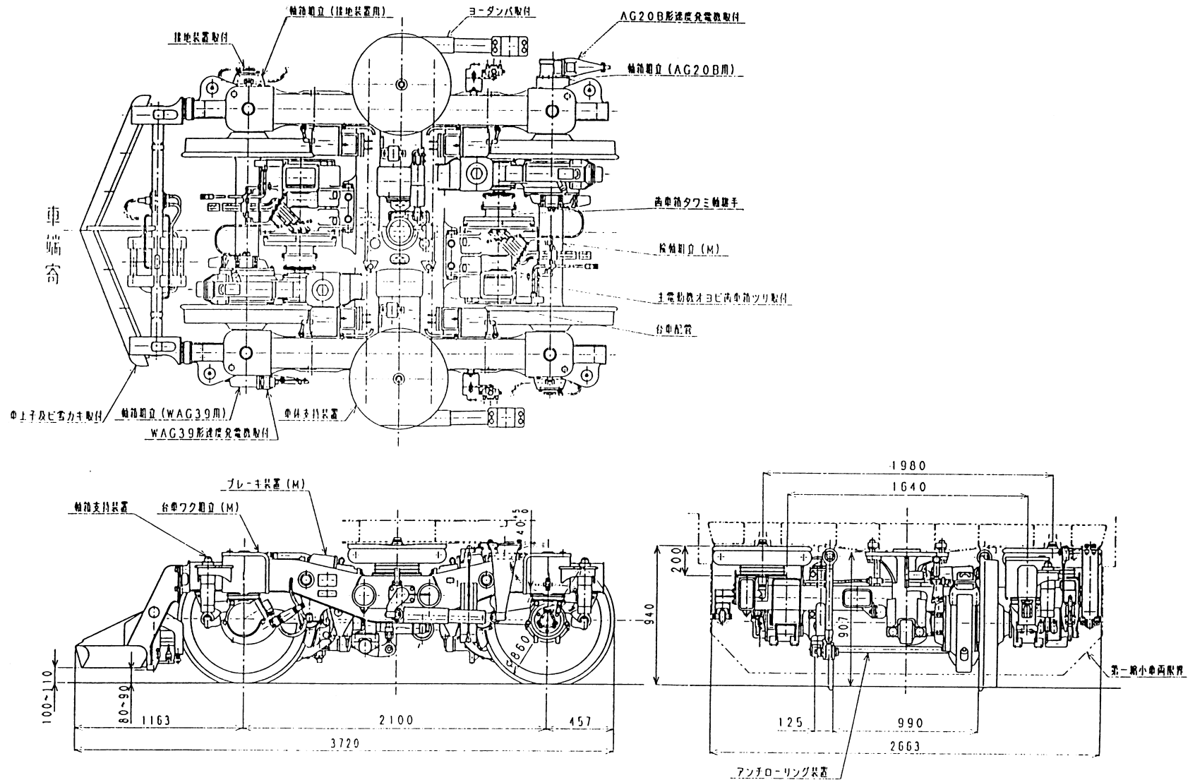
図 17 電動台車 (WDT 59)
