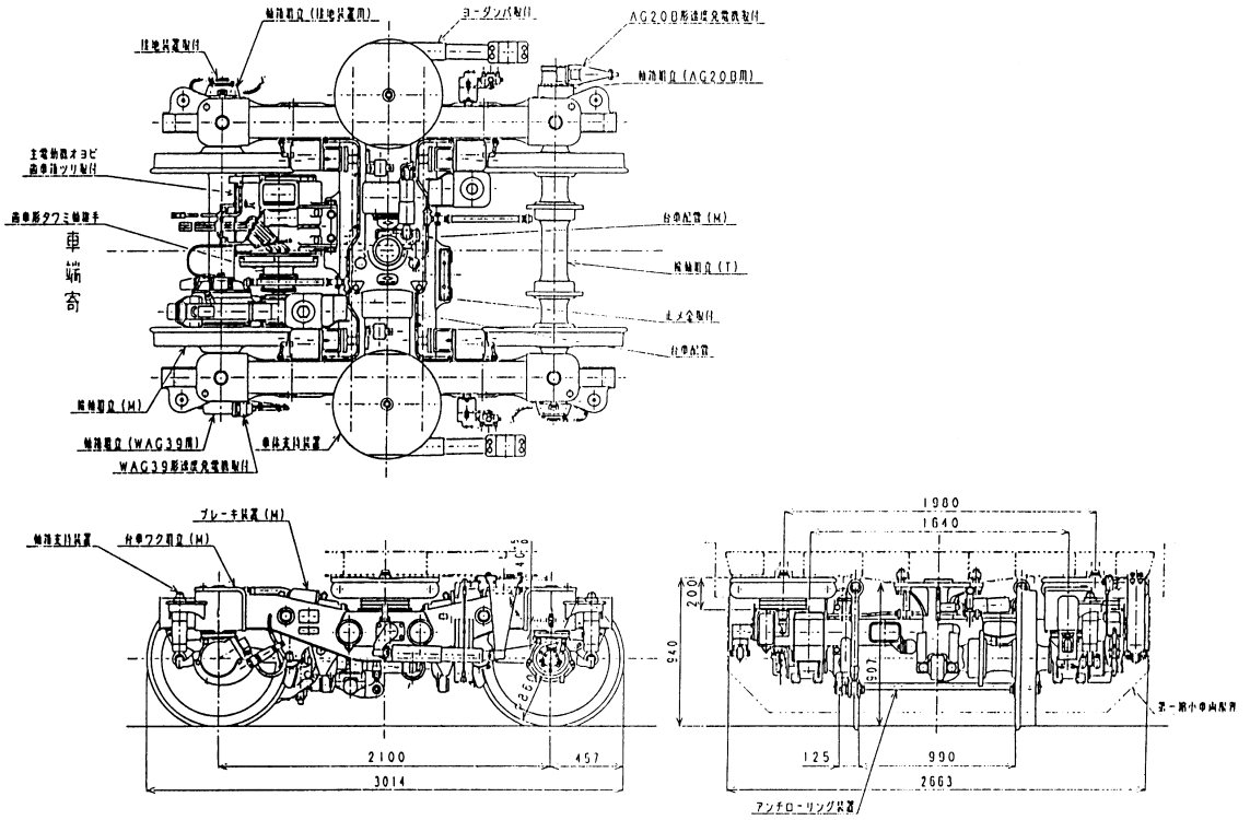
図 18 電動台車 (WD T 59) 3000 代後位台車
