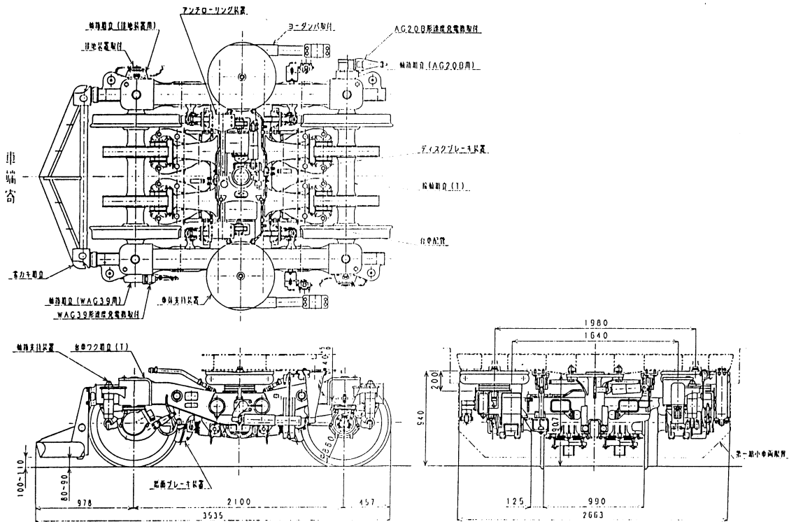
図 19 附随台車 (WTR 243)
