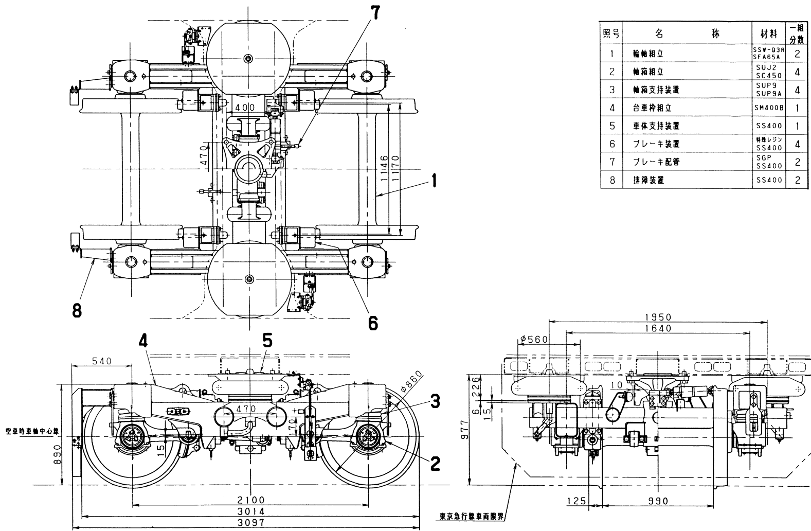
図 12 T台車組立
